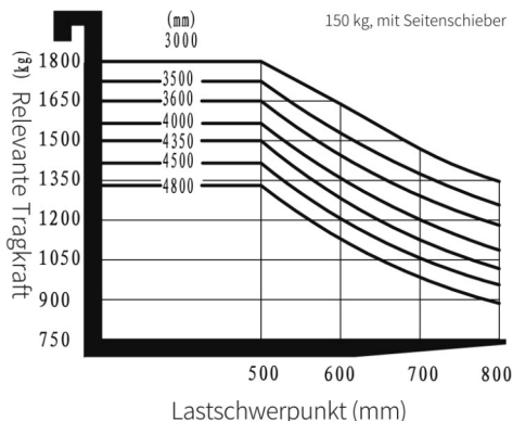
Hublastdiagramm
