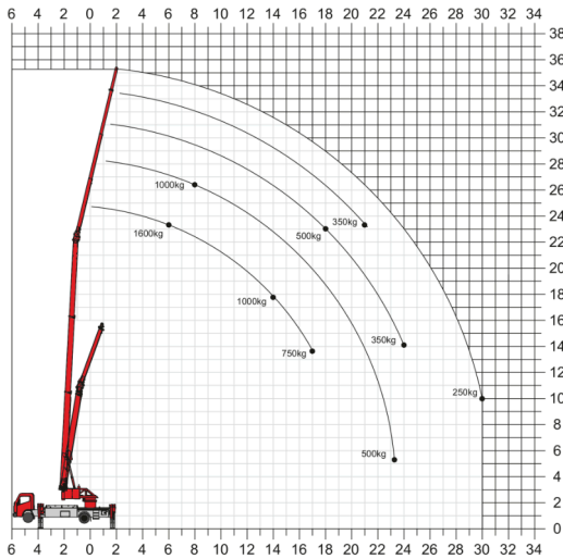
Lastdiagramm Hakenbetrieb
