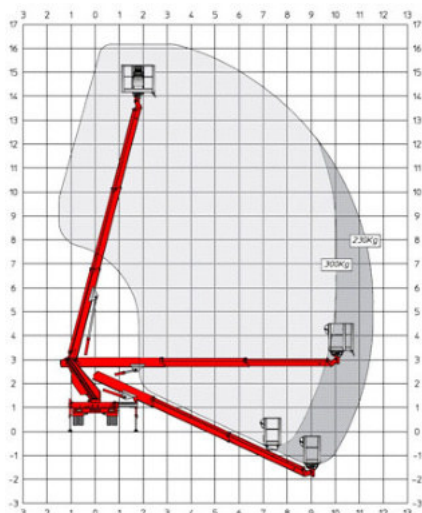
Arbeitsdiagramm
