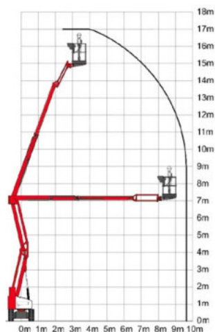
Arbeitsdiagramm
