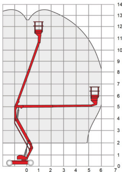
Arbeitsdiagramme
