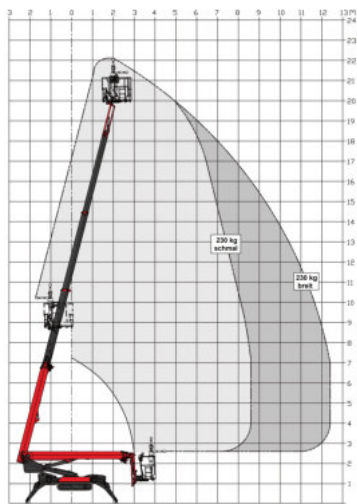
Arbeitsdiagramm
