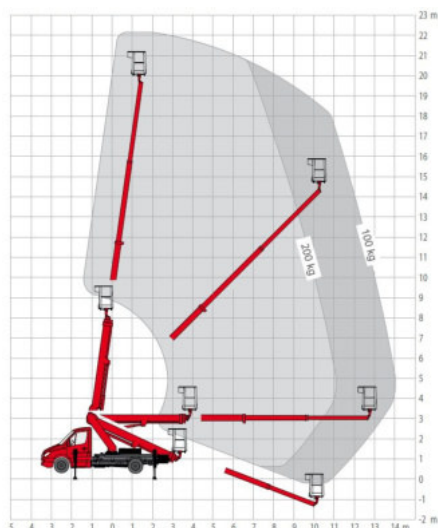
Arbeitsdiagramm
