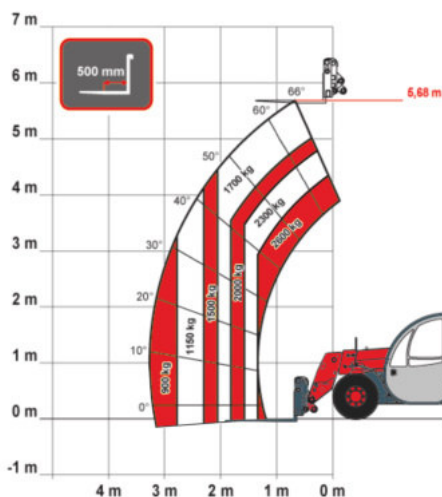
Hublastdiagramm
