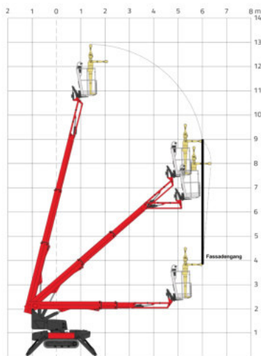
Arbeitsdiagramm
