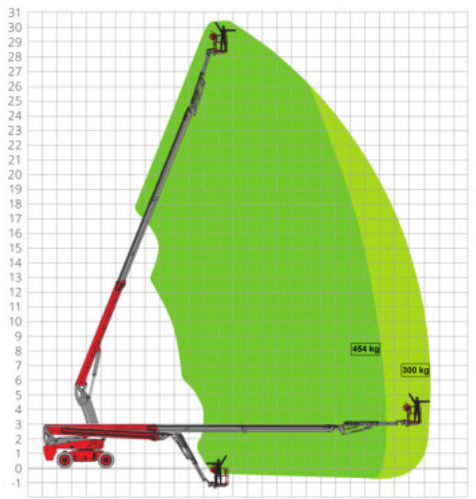
Arbeitsdiagramm
