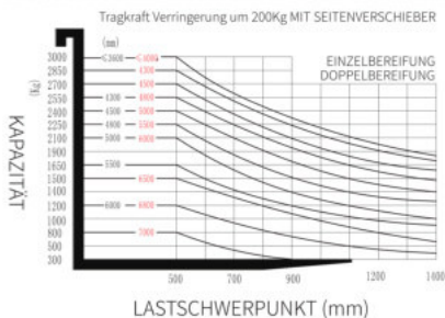
Hublastdiagramm
