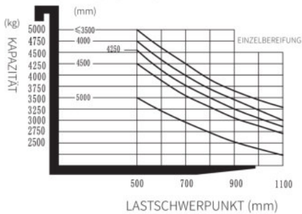
DIAGRAMM DER NENNKAPAZITÄTEN UND LASTSCHWERPUNKTE
