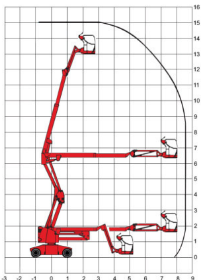
Arbeitsdiagramm
