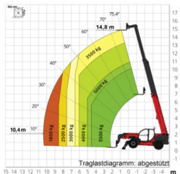
Traglastdiagramm mit Abstützung
