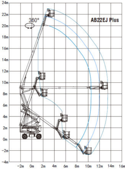
Lastdiagramm
