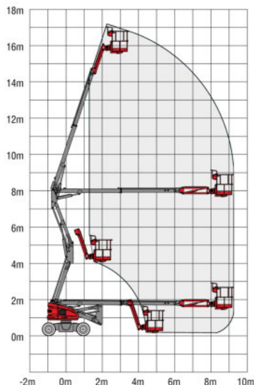
Arbeitsdiagramm
