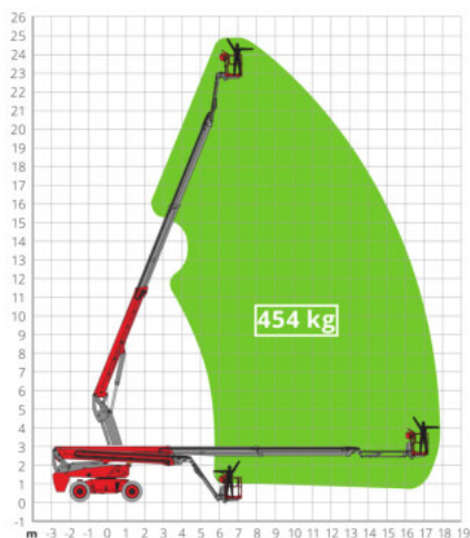
Arbeitsdiagramm
