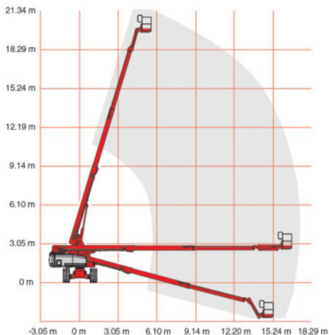
Arbeitsdiagramm
