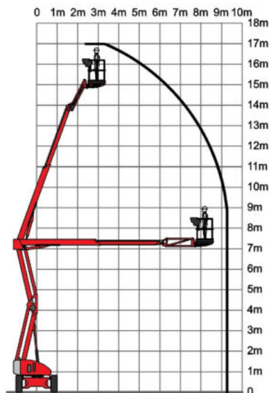
Arbeitsdiagramm
