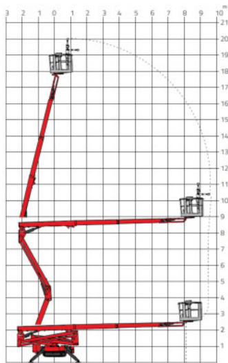
Arbeitsdiagramm
