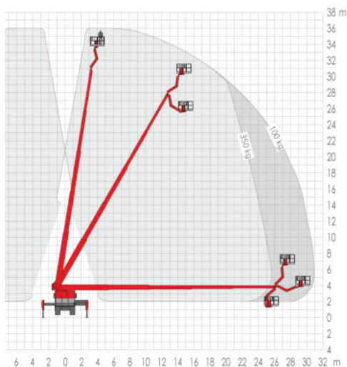
Arbeitsdiagramm
