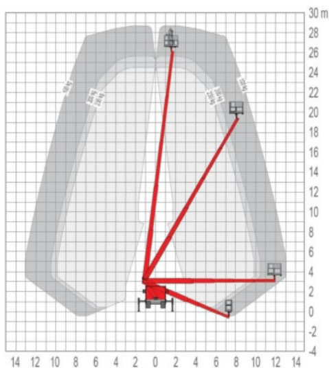
Arbeitsdiagramm
