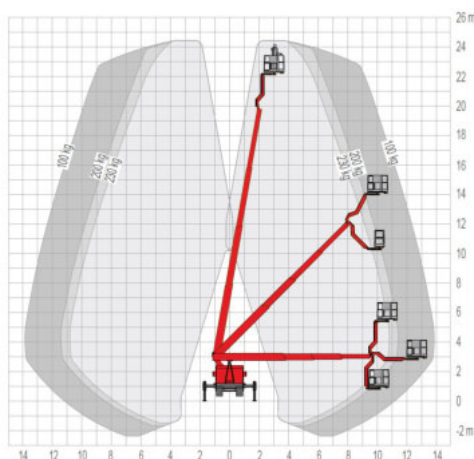
Arbeitsdiagramm
