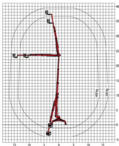
Arbeitsdiagramm
