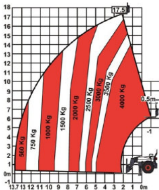
Hublastdiagramm mit Abstützung
