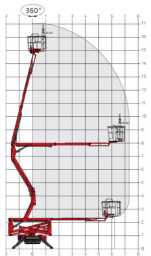
Arbeitsdiagramm
