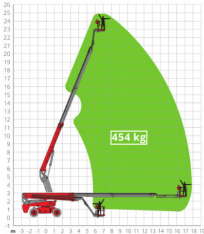
Arbeitsdiagramm
