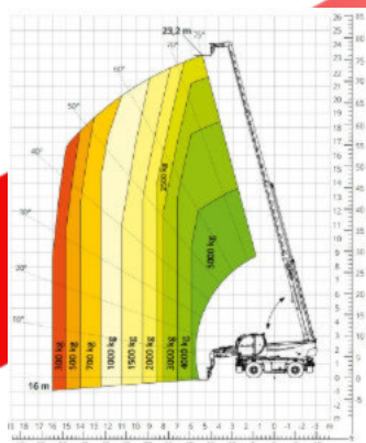
Traglastdiagramm ohne Abstützung
