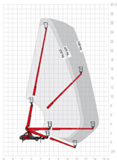
Arbeitsdiagramm
