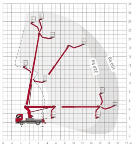
Arbeitsdiagramm
