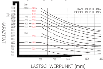
Hublastdiagramm
