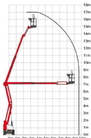
Arbeitsdiagramm
