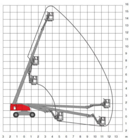
Arbeitsdiagramm
