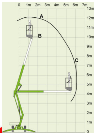
Lastdiagramm
