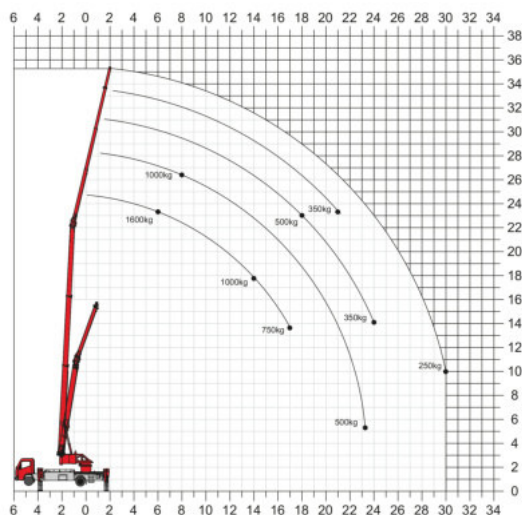
Lastdiagramm Hakenbetrieb
