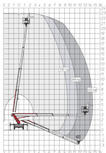
Arbeitsdiagramm
