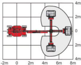
Arbeitsdiagramme
