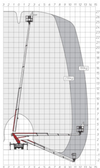
Arbeitsdiagramm
