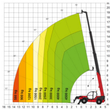
Hublastdiagramm mit Abstützung
