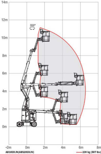
Arbeitsdiagramm
