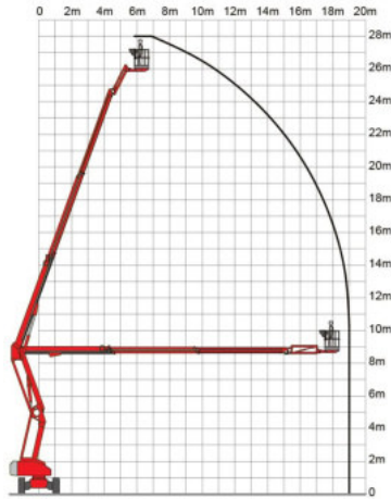
Arbeitsdiagramm
