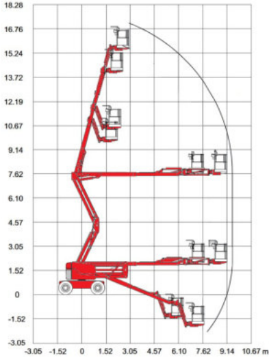
Arbeitsdiagramme
