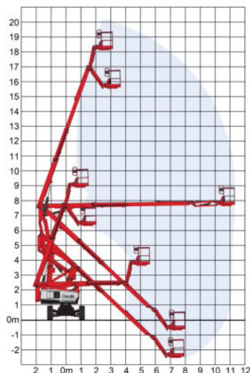
Arbeitsdiagramm
