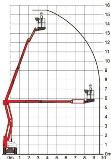
Arbeitsdiagramm
