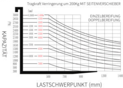
Hublastdiagramm
