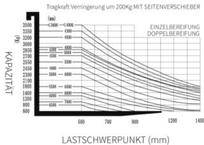
Hublastdiagramm
