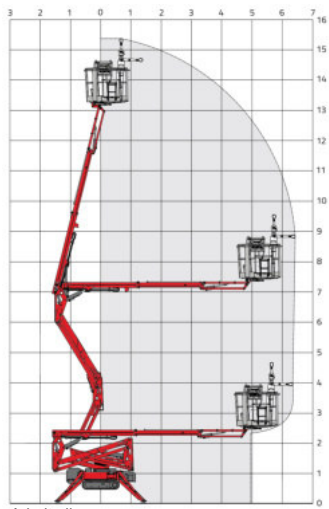
Arbeitsdiagramm
