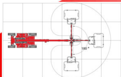
Arbeitsdiagramme
