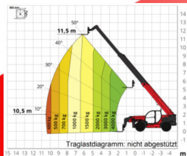
Traglastdiagramm ohne Abstützung
