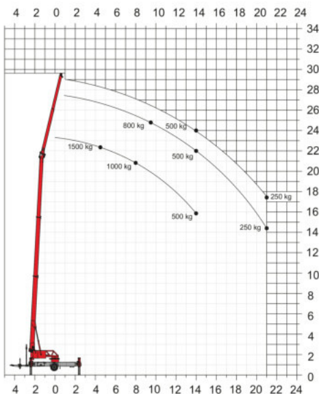
Lastdiagramm Hakenbetrieb
