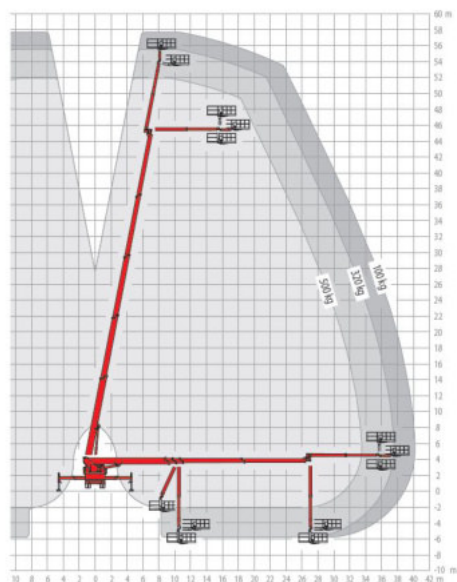
Arbeitsdiagramm
