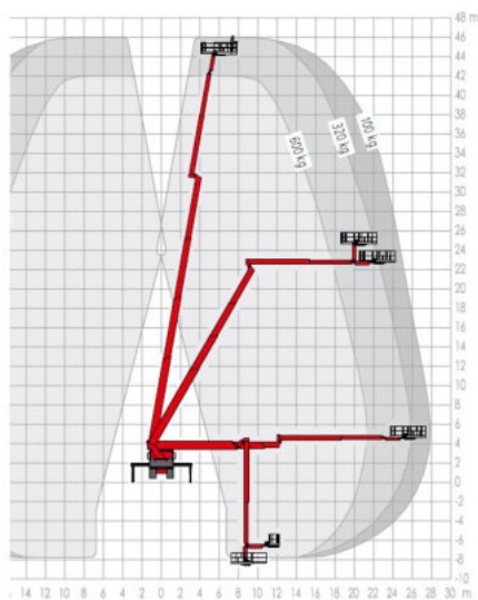
Arbeitsdiagramm
